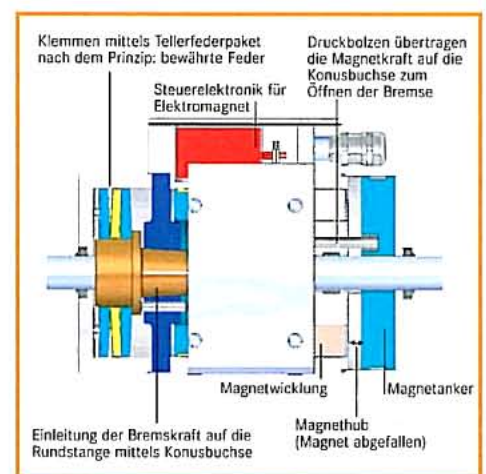
HMSB, Ausführung als Bremse, geklemmt
